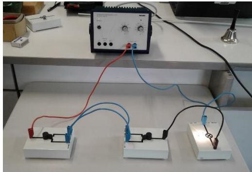
Modell einer Wechselschaltung
